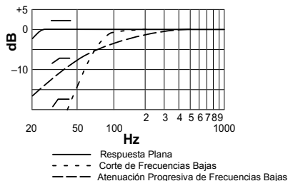
FIGURA 2. RESPUESTAS DE FRECUENCIAS BAJAS
