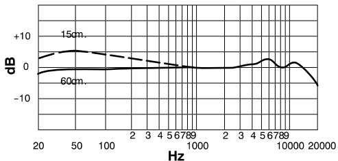
FIGURA 4. RESPUESTA DE FRECUENCIA TIPICA
