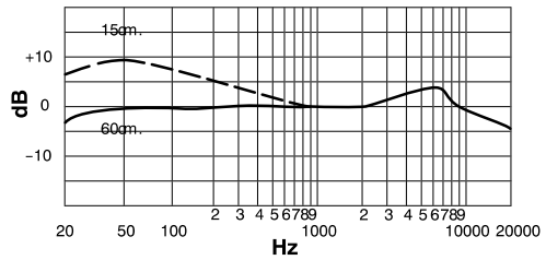
FIGURA 8. RESPUESTA DE FRECUENCIA TIPICA
