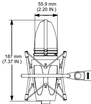
FIGURA 10. DIMENSIONES
