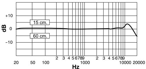
FIGURA 6. RESPUESTA DE FRECUENCIA TIPICA
